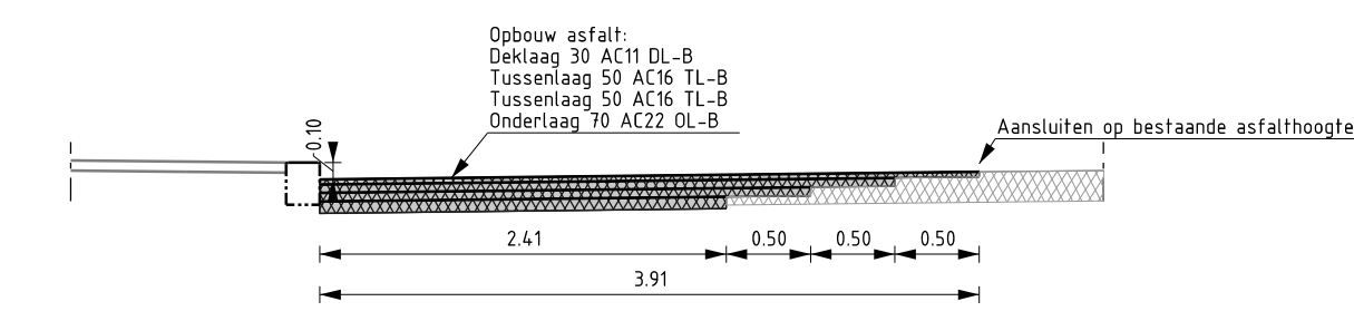
Nieuw DRS SCHAAL 1 : 50
