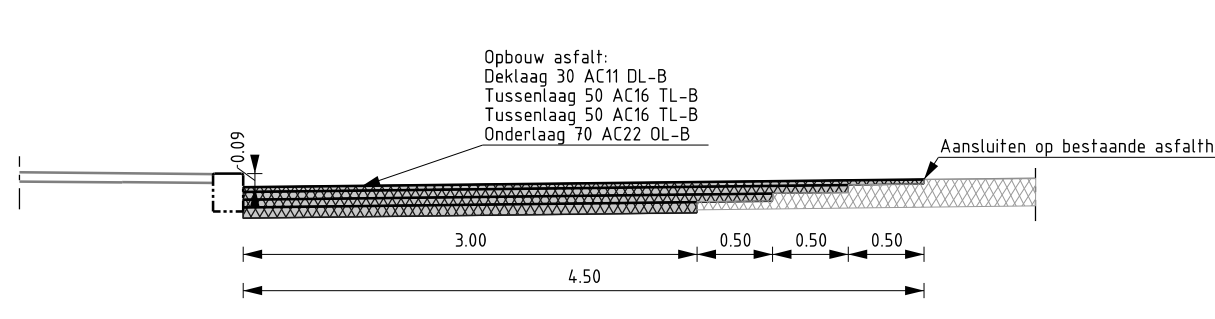
Principe Nieuw (op bestaande puinfundering) SCHAAL 1 : 50
