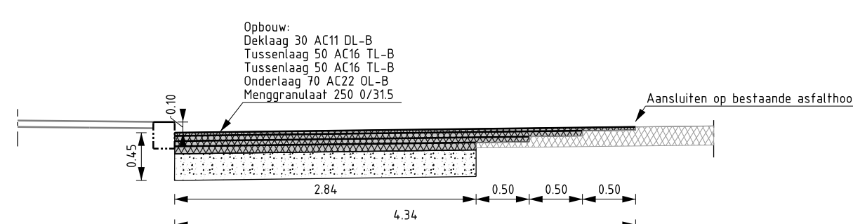
Principe Nieuw (Met aanbrengen menggranulaat) SCHAAL 1 : 50
