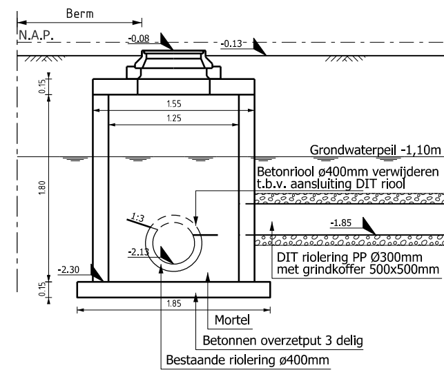
Detail hondehokput Schaal: 1:50
