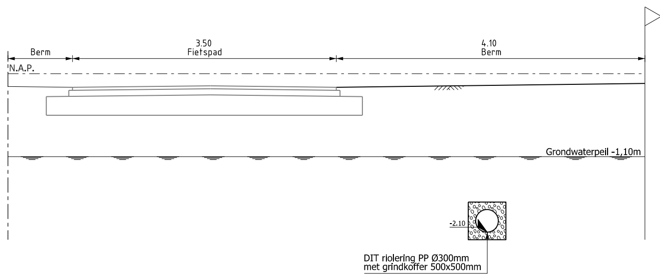
DOORSNEDE A-A Schaal: 1:50
