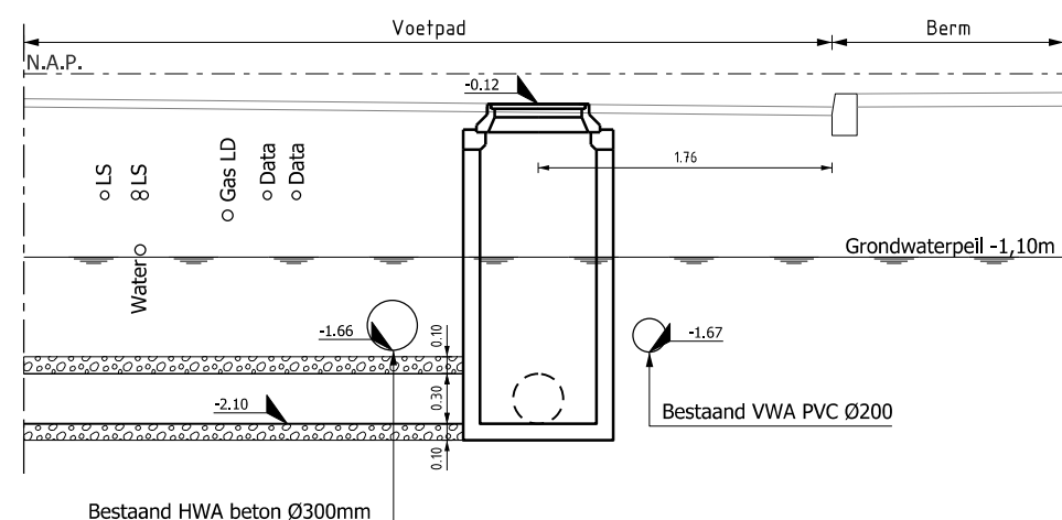
DOORSNEDE B-B Schaal: 1:50
